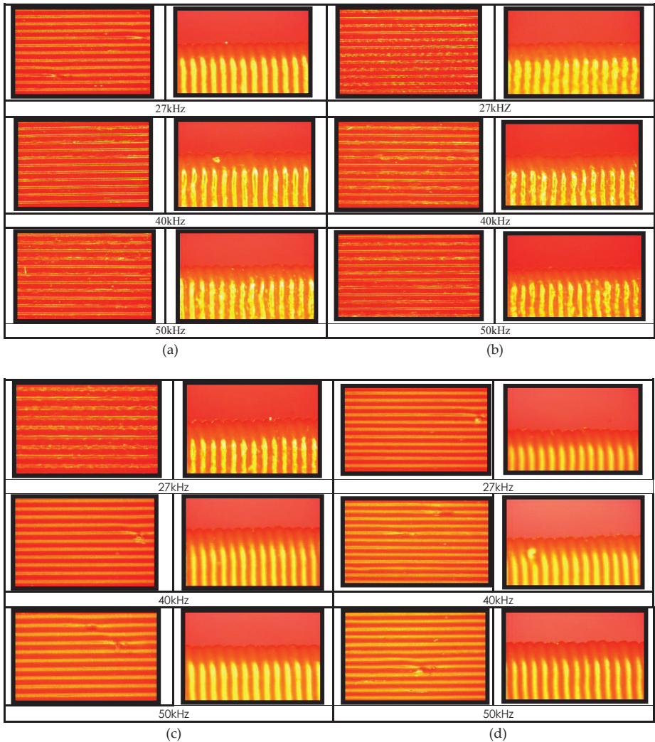
Figure 5: Surface roughness point (a) 1 piezoelectric, (b) 2 piezoelectrics, (c) 3 piezoelectrics and (d) 4 piezoelectrics
